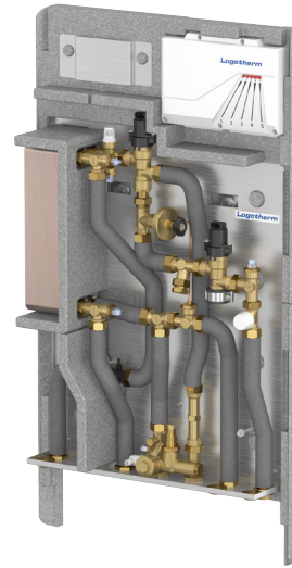
Fig. 6: LogoMatic G2 UC-DHWC-SI
