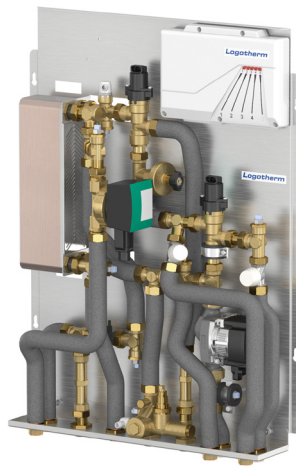
Fig. 5: LogoMatic G2 MC-UC-DHWC-F/S
