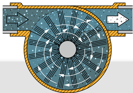
Séparateur conventionnel avec écoulement complet : séparation d'à peine 25% par cycle.
