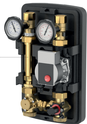
MeiFlow Top S - MC-M Pumpengruppe mit Zählereinbaustrecke mit Metering, EED ready
