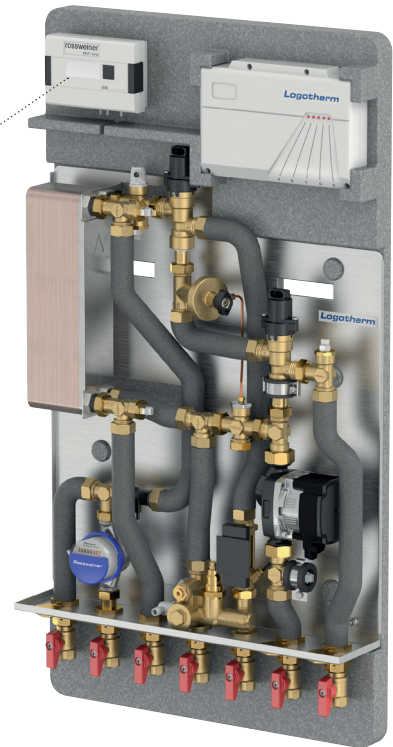
LogoMatic G2 Logotherm® - dezentrale Wohnungsstationen mit Metering, EED ready
