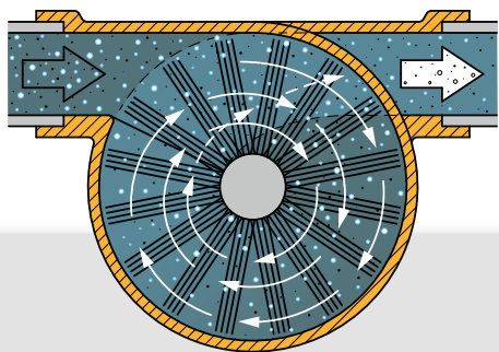
Vanlig separator med fullständigt genomflöde: separerar högst 25 procent per driftcykel.
