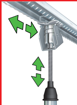
3. Steek draadeind in de unit en schuif deze naar de gewenste positie. Zolang de unit niet gesloten is kunt u deze vrij blijven verschuiven en de hoogte variëren.
