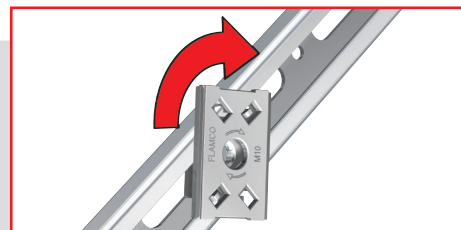
Draai de ClickFit 45°.
