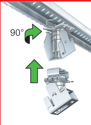
2. Plaats de FlamcoFit unit in de rail en draai deze in positie. De unit kan nu niet meer uit de rail vallen.
