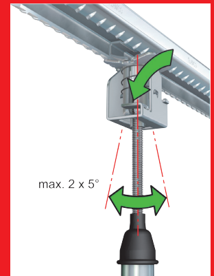
5. De FlamcoFit unit heeft een axiale bewegingsruimte van 2 x 5°.
