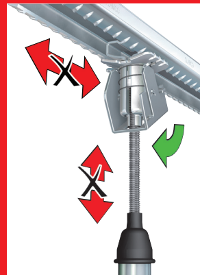
4. Sluit de unit. Nu is de positie in de rail en de hoogte van de buis vergrendeld.
