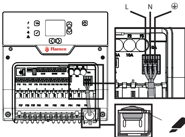
Anslut strömkabeln (100–240 V AC ~1N PE, 50/60 Hz)
