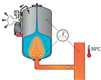
2. Opvarmning Vandmængden og systemtrykket øges. Enheden reagerer på dette ved at åbne den magnetventilen. Vand strømmer ind i beholderen.
