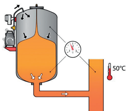
4. Nedkøling Vandmængden og systemtrykket aftager. Kompressoren øger trykket i luftrummet, vand overføres tilbage i systemet. Dette genopretter det ønskede systemtryk.
