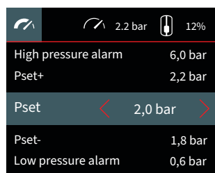
Schermata impostazioni
