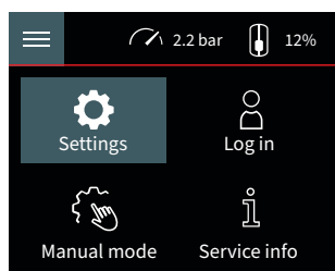
Schermata menu
