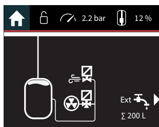
Schermata operativa
